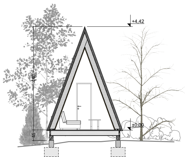
presjek
