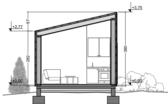
presjek
