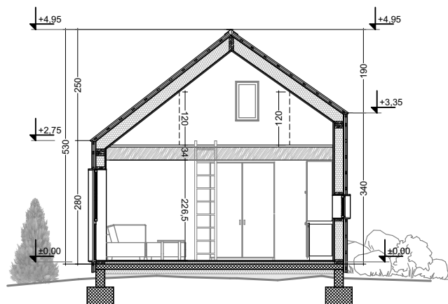
presjek
