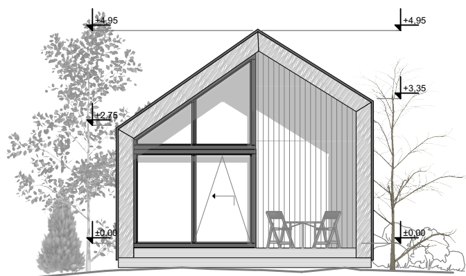
fasada 1
