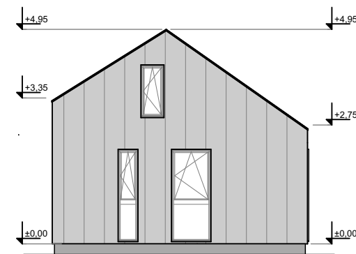
fasada 2
