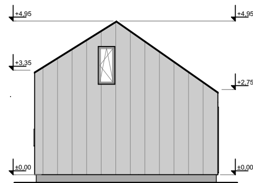
fasada 2
