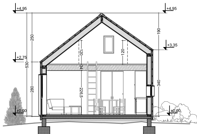
presjek
