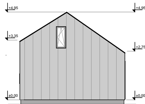
fasada 2
